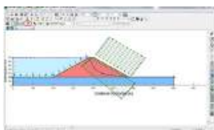
Figura 1: Software Geostudio
